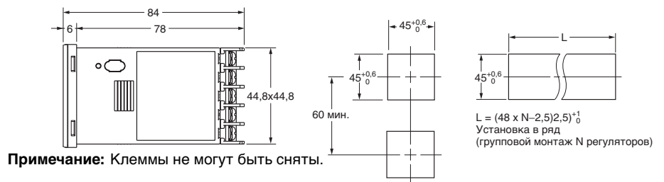
Размеры монтажного выреза
